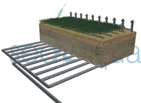
HUMEDALES CONVENCIONALES DEPURACIÓN ECOLÓGICA
